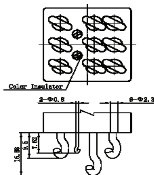
Pin Form: 4
